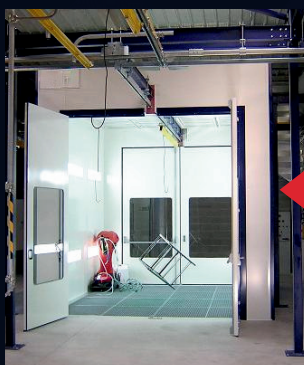
Cabine de poudrage
